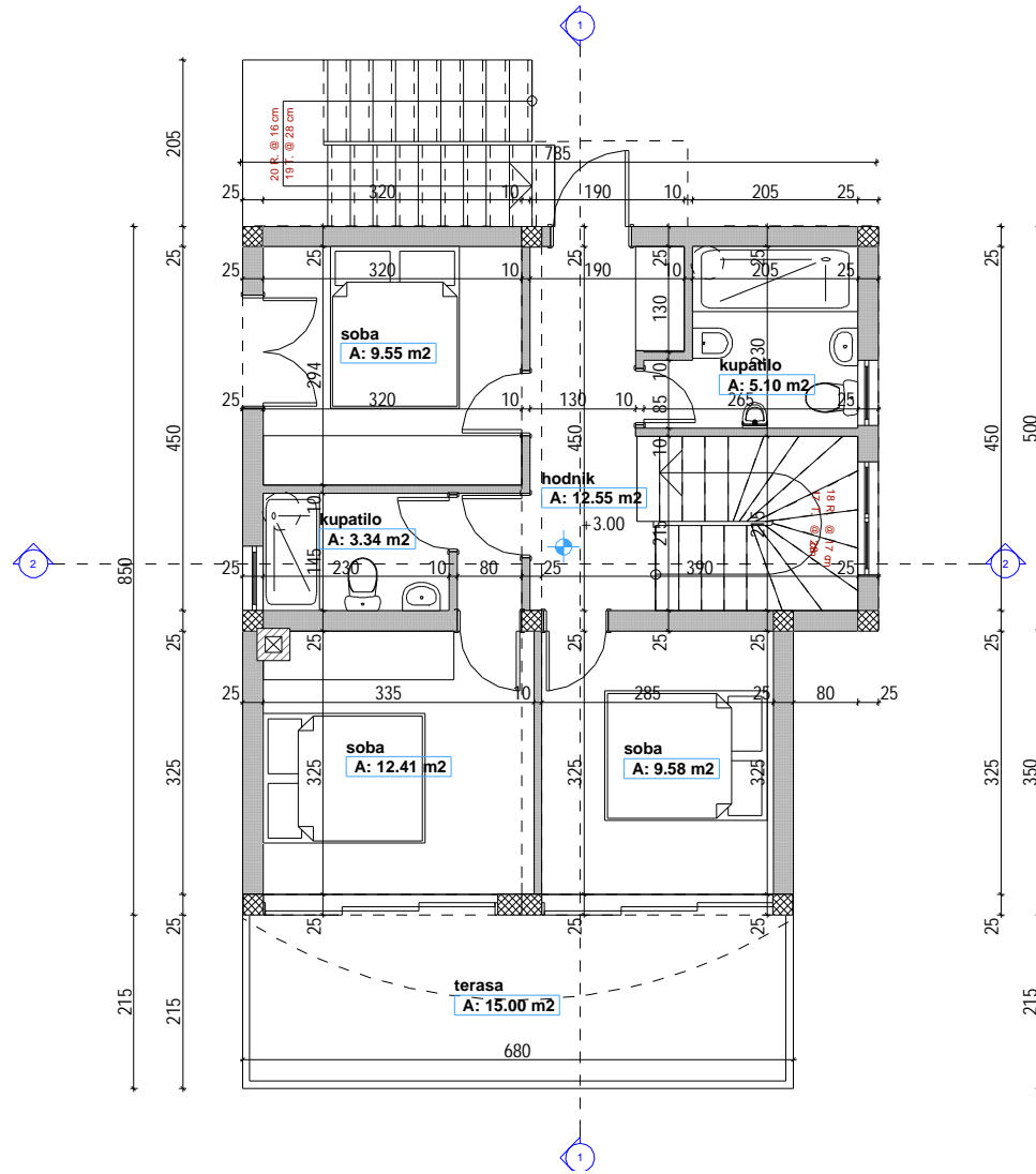
osnova sprata m 1:100
