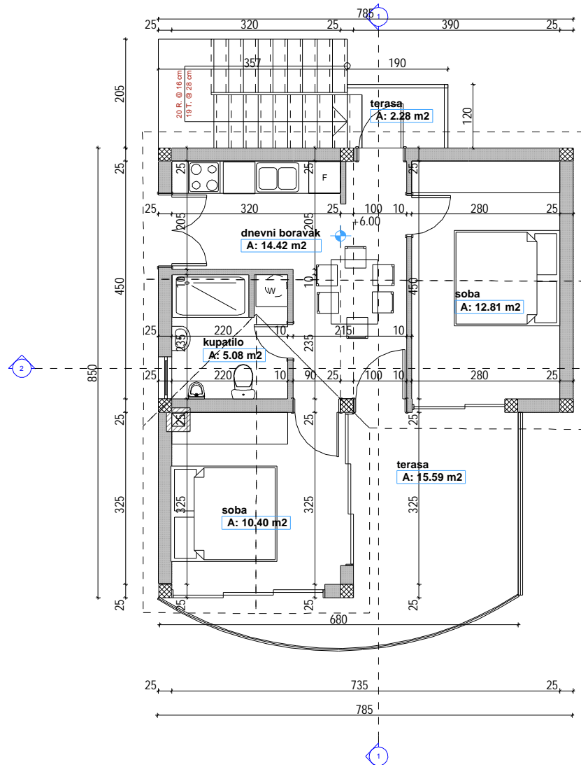
osnova potkrovlja m 1:100
